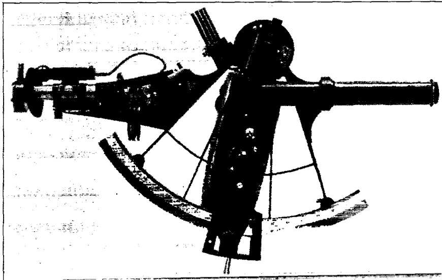
FIG. 13 —Fischer sextant
