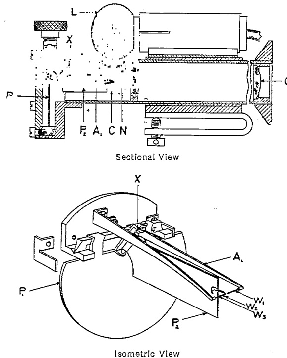
FIG. 14.—Fischer pendulum horizon
