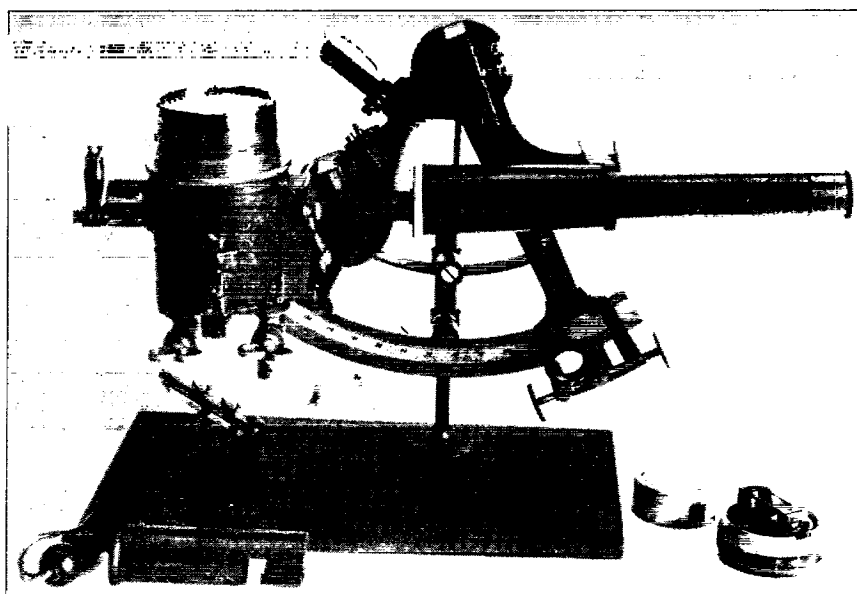
FIG. 15.—Fleuriais sextant
