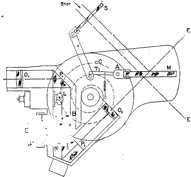
FIG. 12.—R. A. E. sextant, diagram
