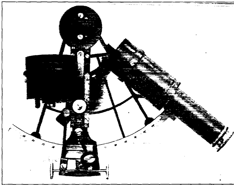
FIG. 16.—Derrien sextant
