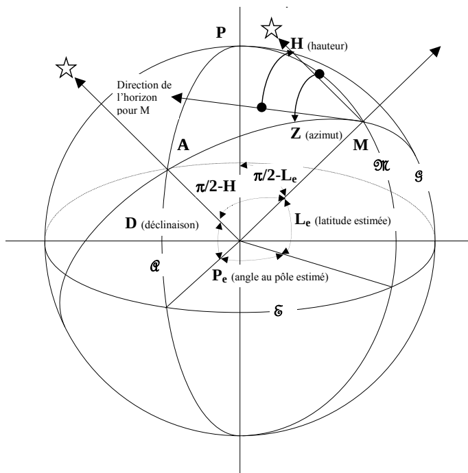
6 : Application au triangle de position sur un globe terrestre. La figure en perspective déforme l'orthogonalité en M de la verticale et de la direction de l'horizon. Cette orthogonalité existe toutefois et il en résulte que l'arc AM a pour mesure \pi/2-H .
