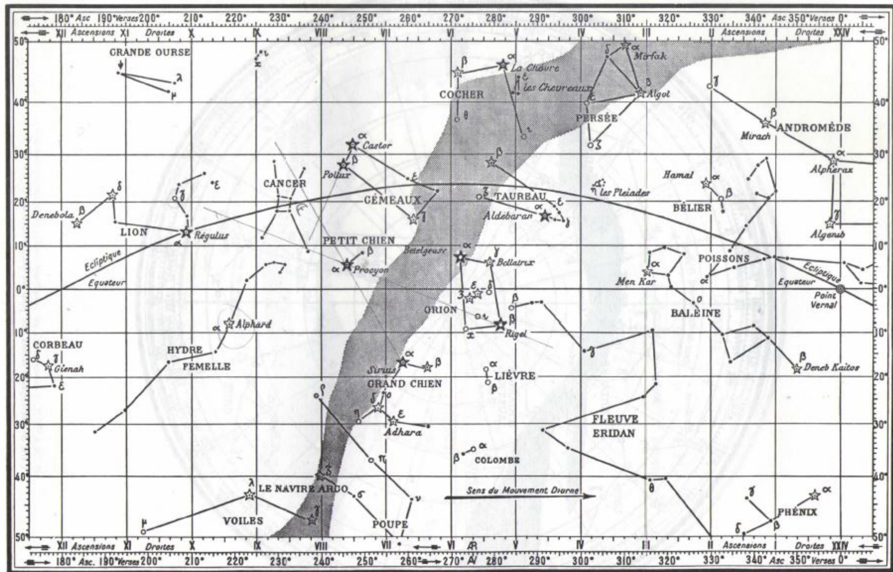
Carte équatoriale du ciel (Mercator), de 50° N à 50° S en Déclinaison et de 0 h à XII h en Ascension droite.
